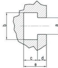
2 Detail (T-slot)
